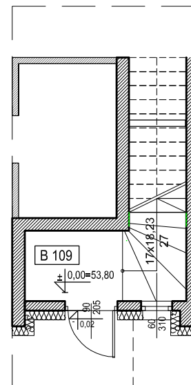
FRAGMENT RZUTU PARTERU Z WEJŚCIEM DO LOKALU 2
